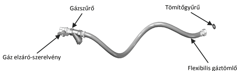
5. ábra: Csatlakoztatás flexibilis tömlővel (opció, a készülék gyártónál megvásárolható)
