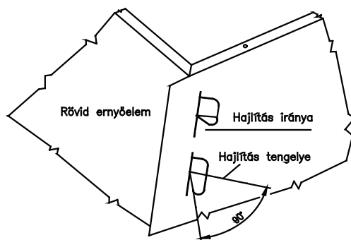
3.ábra: Ernyők összeszerelése
