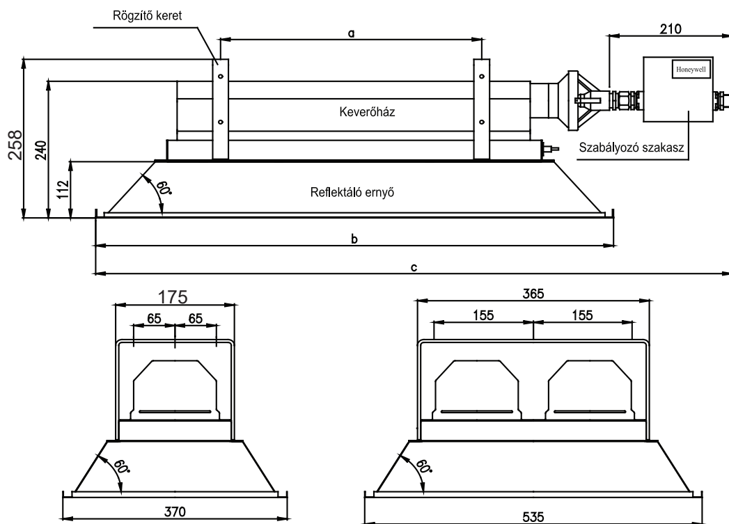
2. ábra: Gázinfra hőszugárzók jellegrajza
